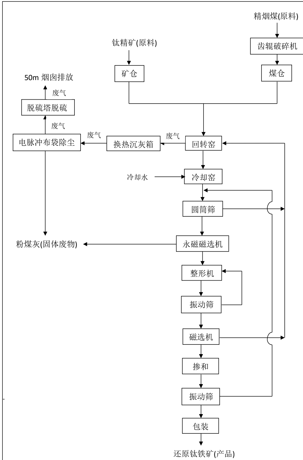
图2 工艺流程图
